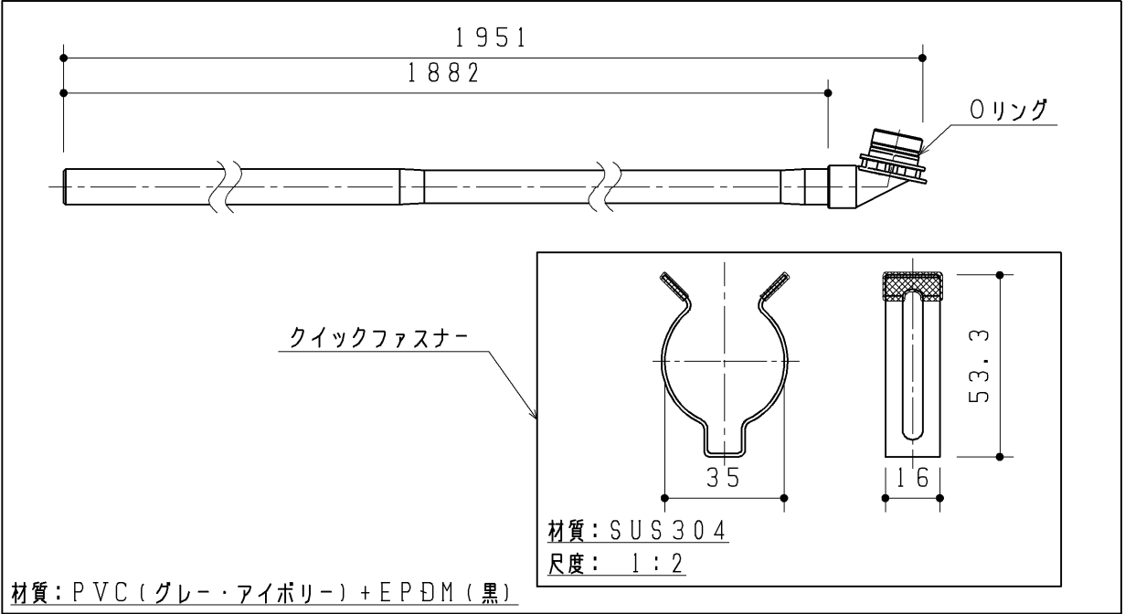
排水管組品
