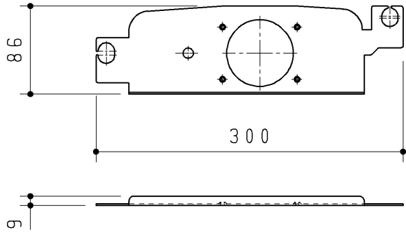
材質：SGHCまたはSGCC
