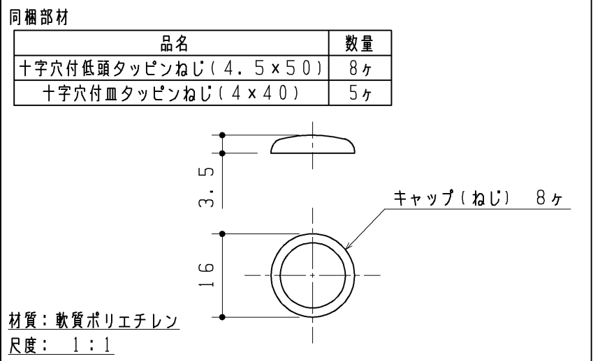
ねじセット
