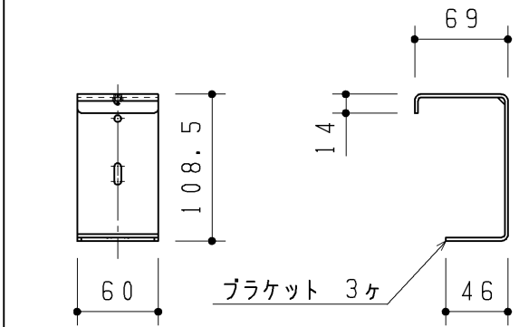
材質：SGHCまたはSGCC
