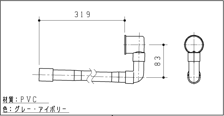
排水管組品
